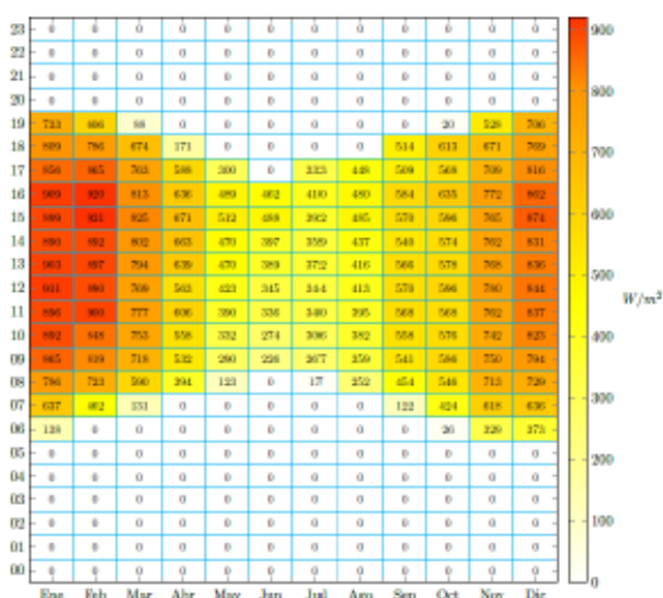
Promedio para la radiación directa normal para cada hora y mes
